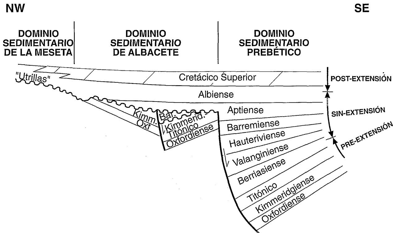
Figura 2.- Modelo tectonosedimentario con las características estratigráficas y relaciones espaciales de cada dominio sedimentario. (Modificado de Vilas y Querol 1999)
